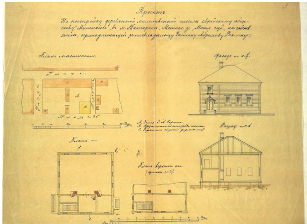
► Малюнак 1. Праект будаўніцтва драўлянай малітоўнай школы «Мішнае» у м. Татарск Мсціслаўскага павета. 1892 год Крыніца: Нацыянальны гістарычны архіў Беларусі.
