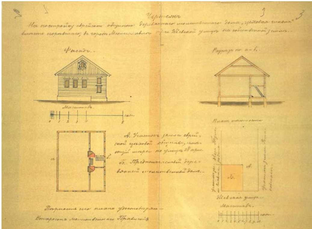
Малюнак 2. Незацверджаны праект узвядзення «Цэхавай школы» ў Мсціславе. 1898 год Крыніца: Нацыянальны гістарычны архіў Беларусі.
