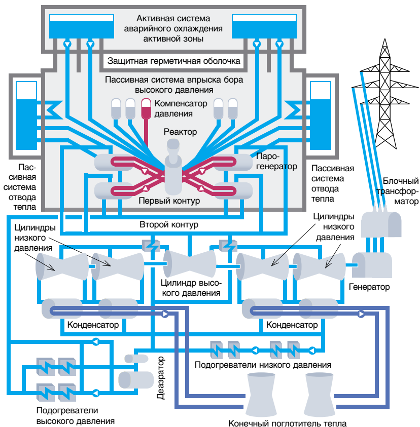
Принципиальная схема энергоблока АЭС-2006
